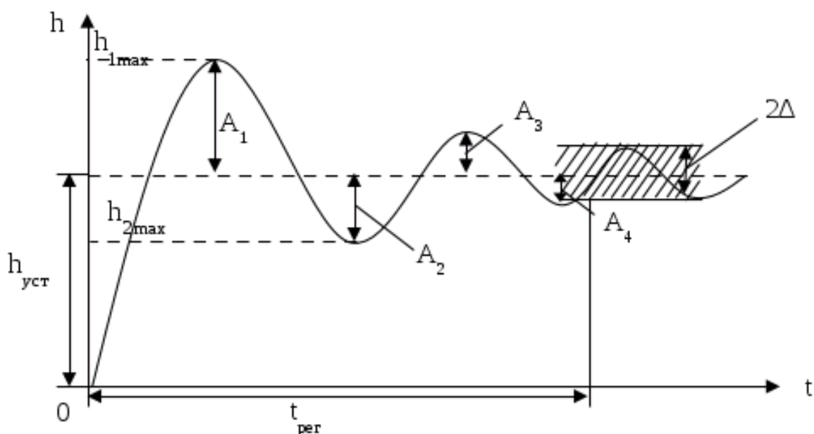
Рис. 1 – Переходная характеристика системы управления
